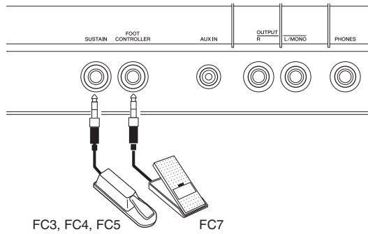
Задняя панель
