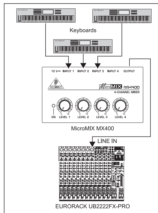
Каблирование MX400
